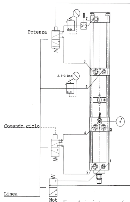
Figura 3_ impianto pneumatico di riferimento
