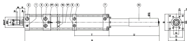
Rysunek 1_Schemat siłownika_WERSJA „E”
