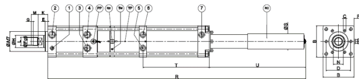
Abbildung 1 _ Schematische Ansicht der Einheit VERSION „E“
