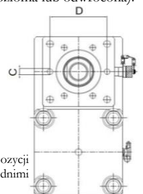
Rys.4_Kołnierz siłownika w pozycji podłużnej z odpowiednimi mocowaniami
