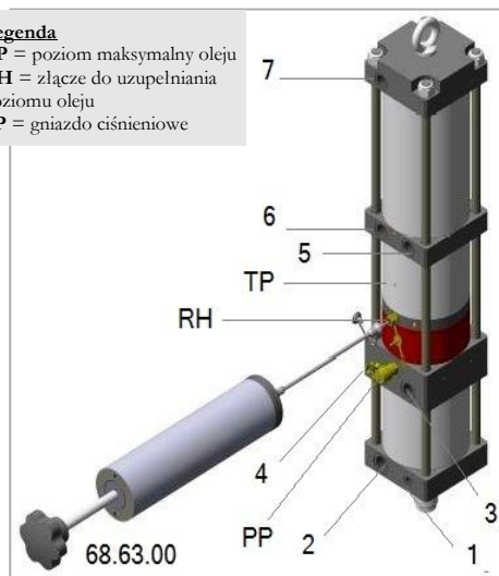
Rysunek 6 _ Podłączenie pompy do uzupełniania oleju
