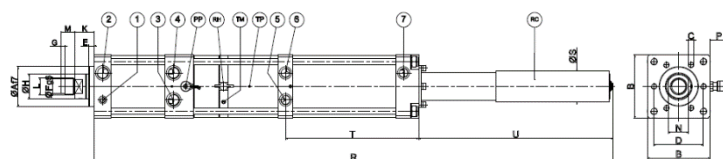
Figura 1 _ vista schematica unità_versione “E”
