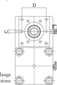
fig.4 Vue de la flange en ligne et ses fixations
