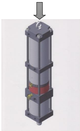
Figure 7 _ Vue avec anneau de levage
