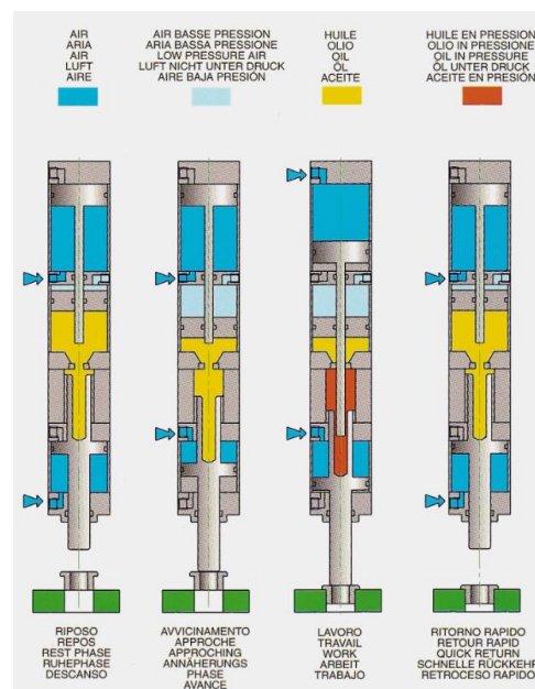
Abbildung 2 _ Betriebsprinzip
